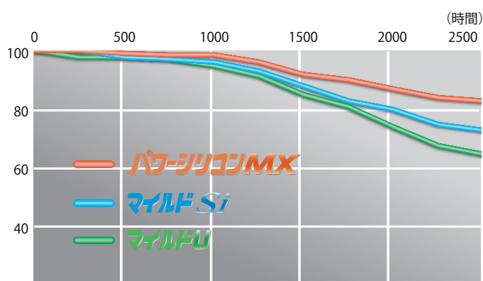
光沢保持率 基材：スレート 試験色：グレー（N4.5程度）
