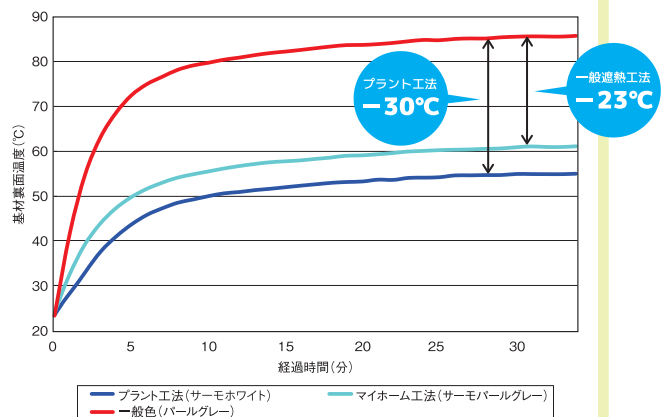
赤外線ランプによる遮熱効果試験結果
